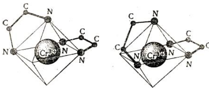
Рис. 71. Схематичне зображення структур дзеркальних ізомерів комплексів хрому з етилендіаміном.
