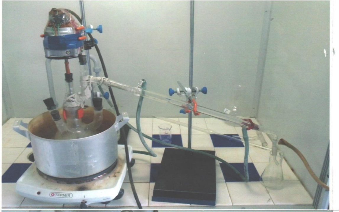
Рис.2. Установа для концентрування смоли
